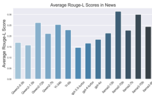
[뉴스(News), 소설(Novel), 등 다양한 텍스트 유형에서 LLM이 원본을 얼마나 충실하게 재현하는지 보여주는 그래프 4)
