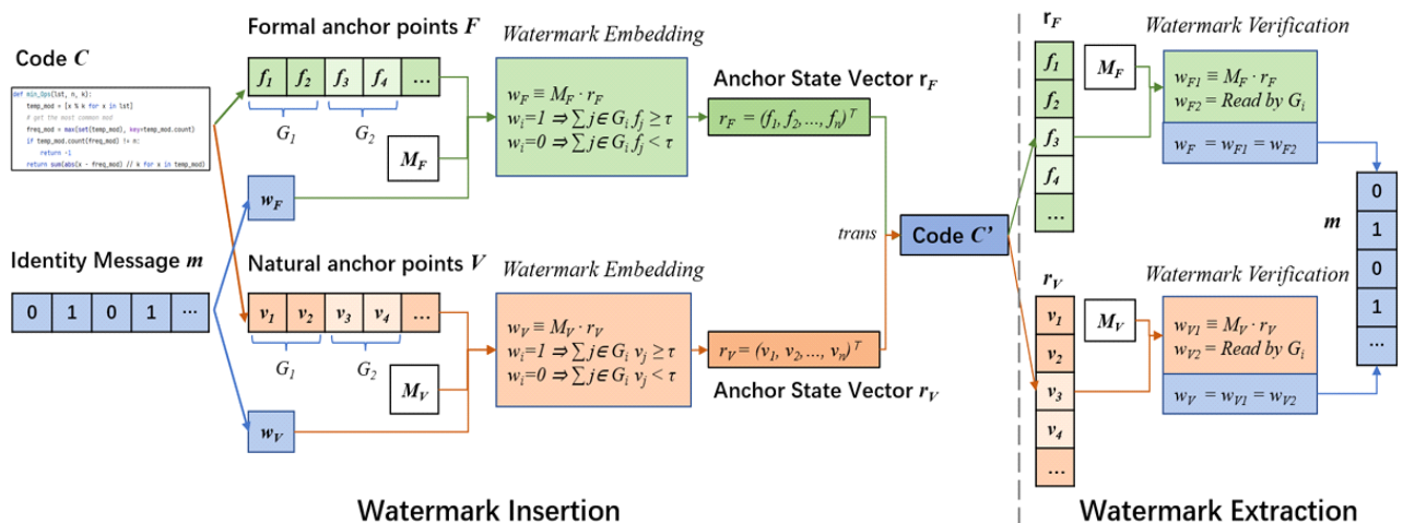
[그림 1] MATRIX의 워터마크 삽입 및 추출 프로세스
